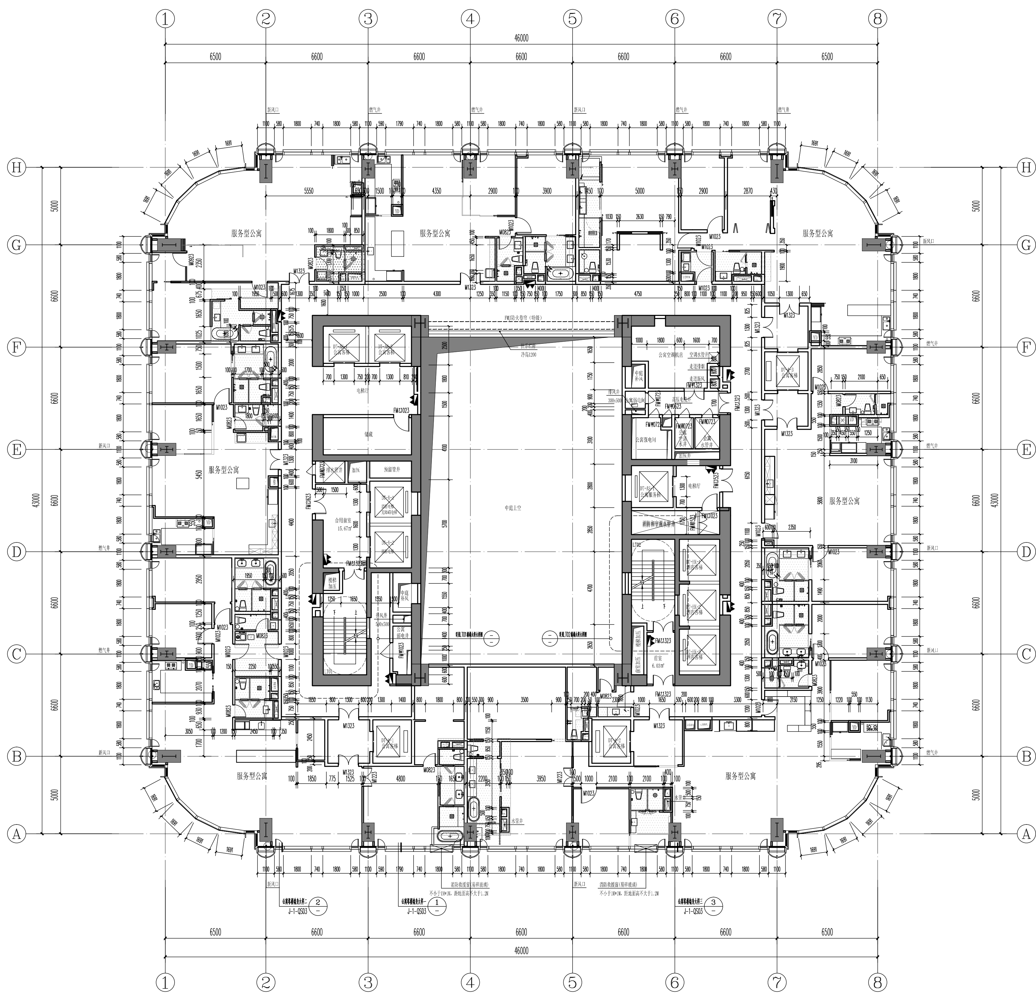
二十八~三十四层平面图 1:150
